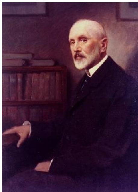
Eötvös Loránd 1848-1919.
